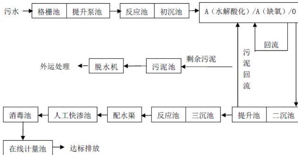
图 5.2-1 扩建 1 万 m 3 /d 处理工艺流程图
