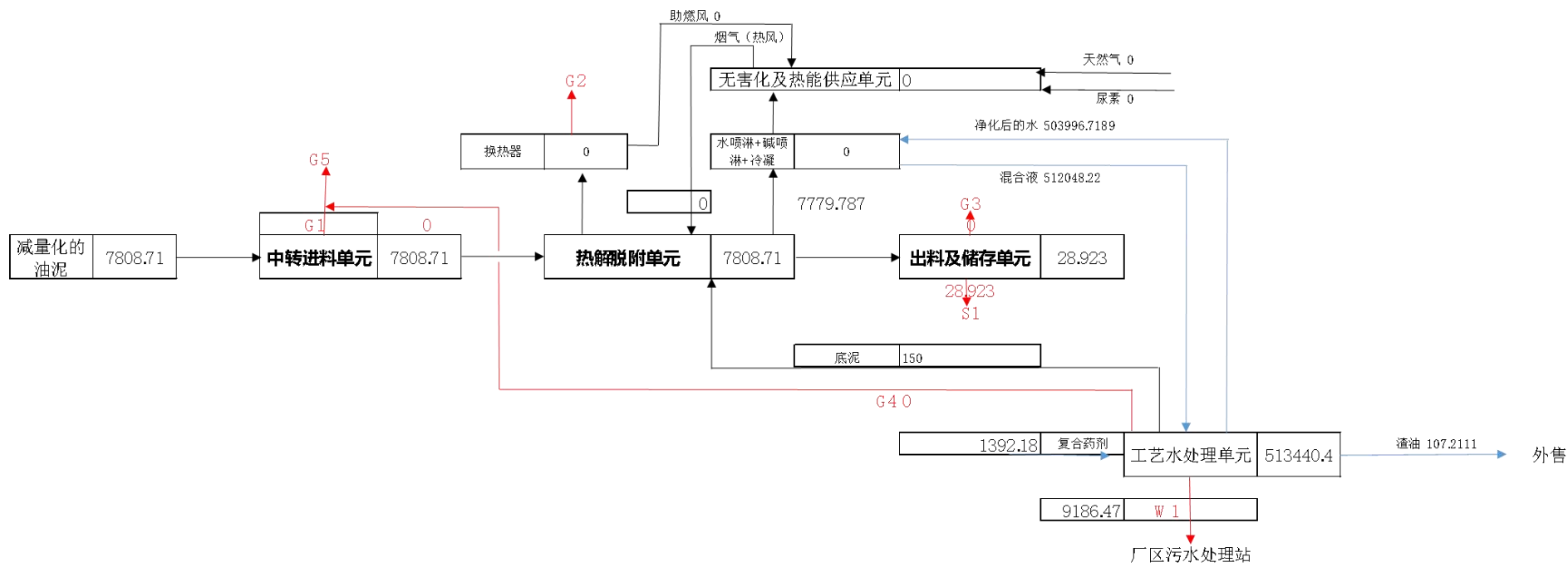
图 3.6-3 本项目技改后水平衡图
