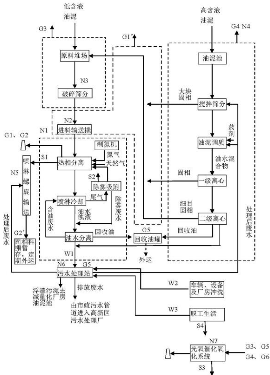
图2.6.1 本项目生产工艺流程及产污环节图
