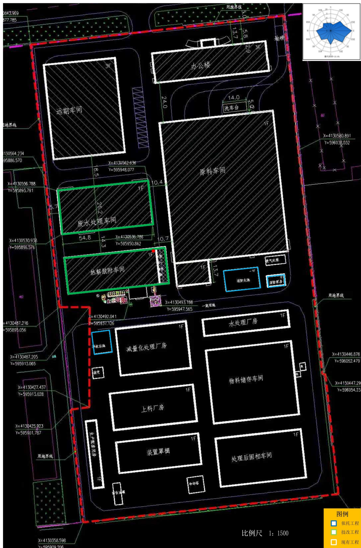
图 3.3-4 本项目厂区平面布置图
