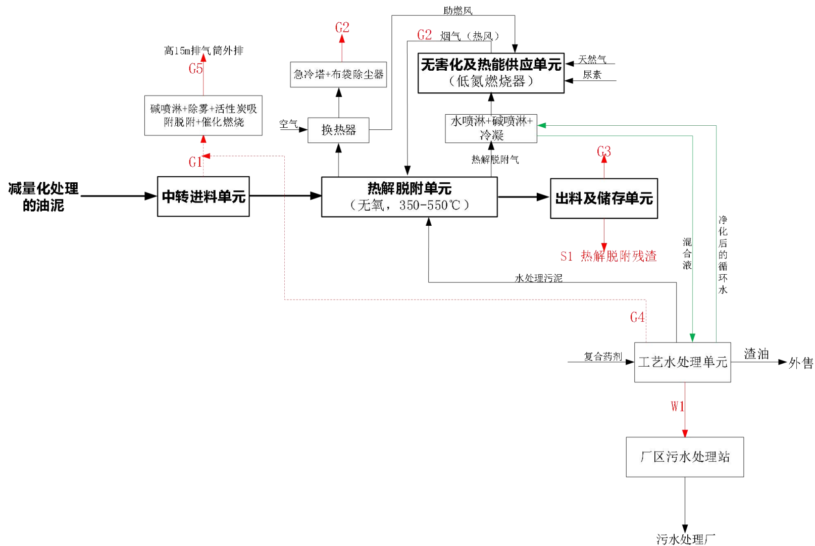
图 3.4-7 本项目装置工艺流程及产排污环节图
