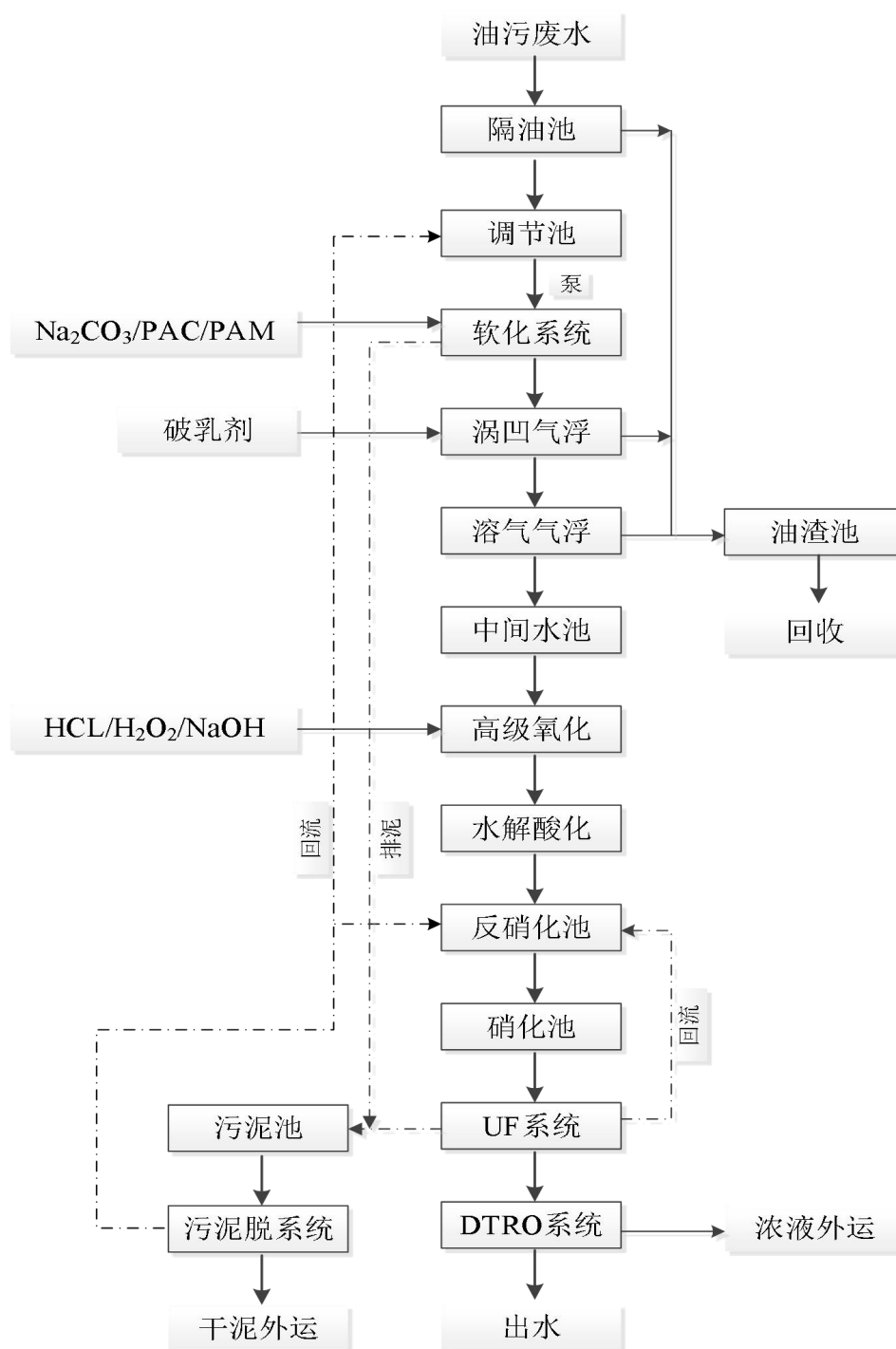
图 3.4-6 废水处理单元工艺流程图
