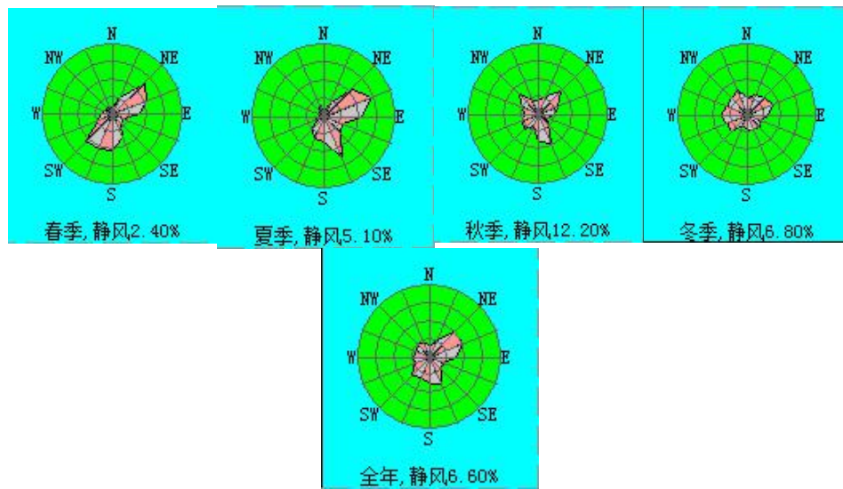
图 5.1-5 2019 年各季与年平均风向频率玫瑰图
