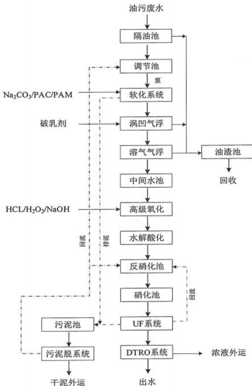
图2.7-2 污水处理工艺图
