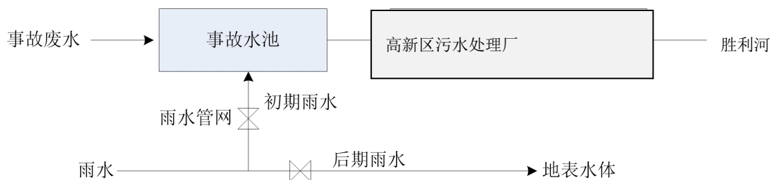
图 7.6-3 拟建项目事故排水控制管线图
