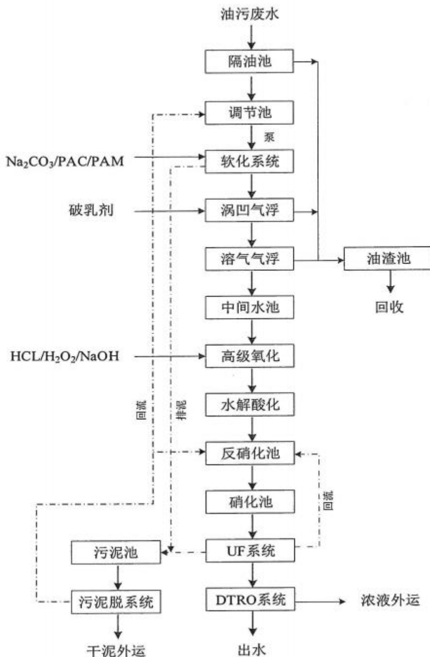
图 3.5-1 污水处理工艺流程图
