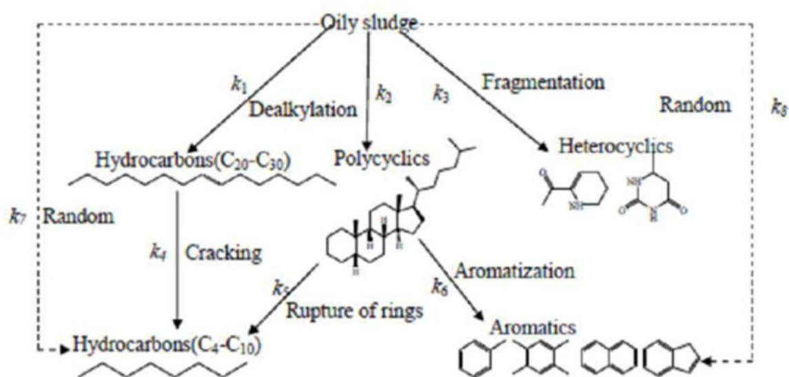
图 3.4-2 油泥砂和含油污泥热解反应路径示意图
