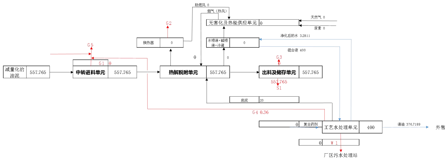
图 3.6-2 本项目油平衡图
