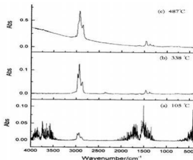
图 3.4-4 油泥在氮气下热解产物 IR 图
