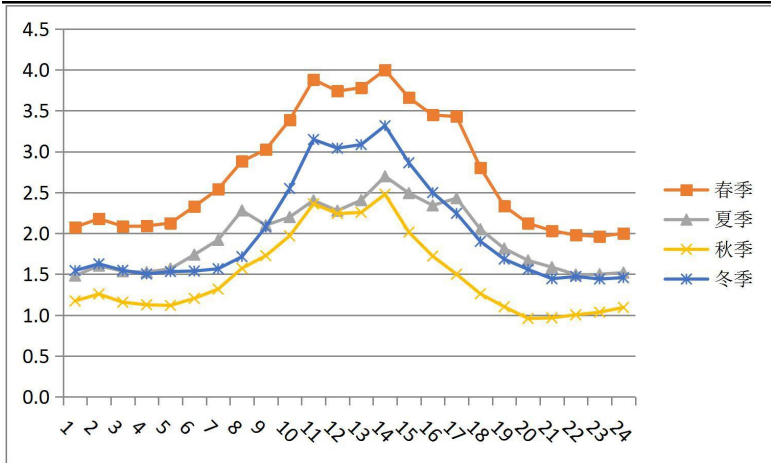
图 5.1-4 2019 年季小时平均风速日变化曲线图
