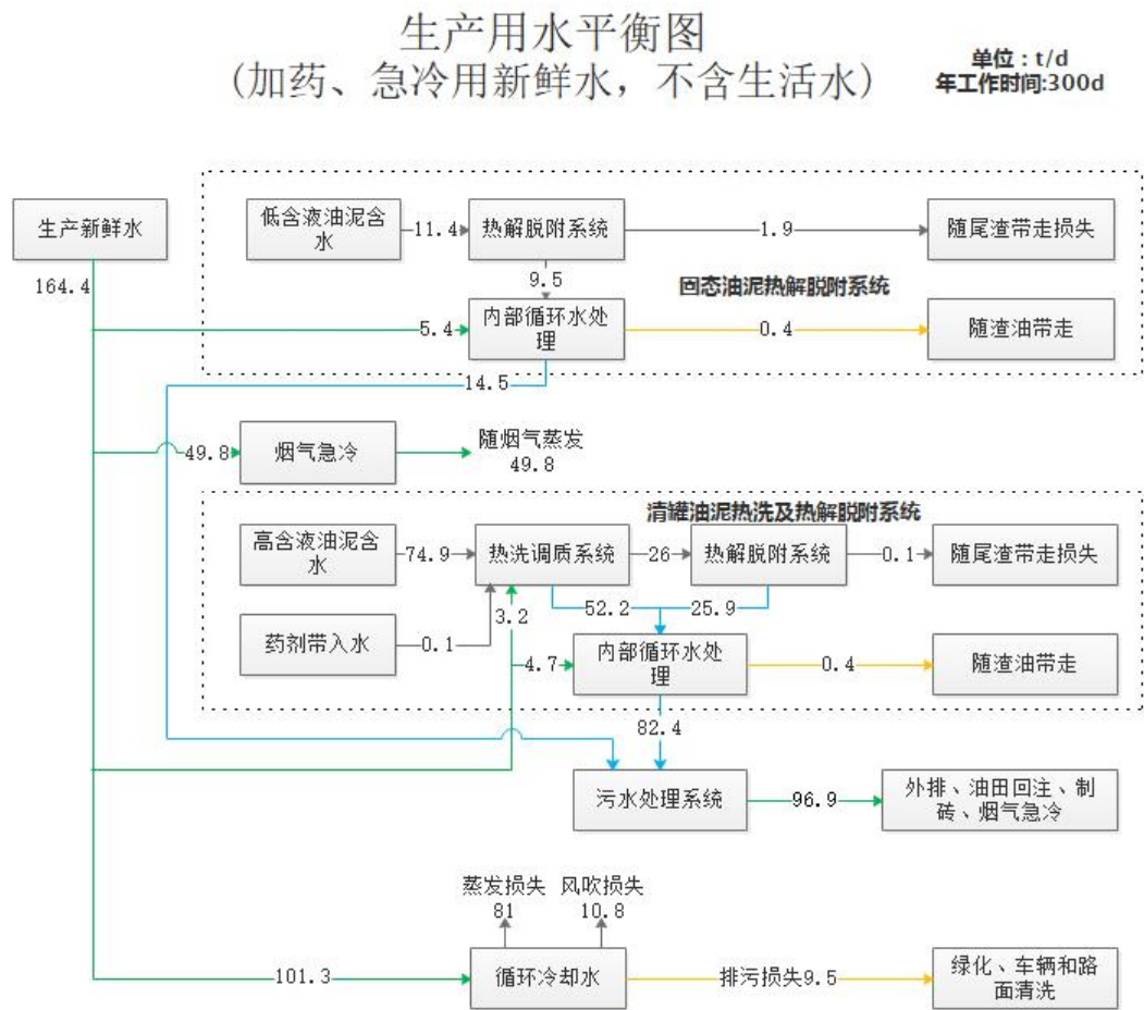
图 3.9-3 本项目水平衡图
