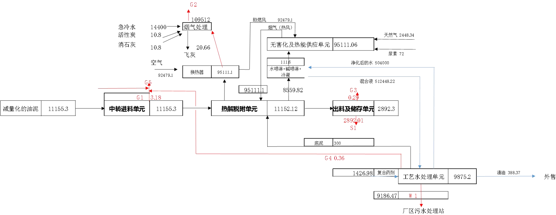
图 3.6-1 本项目技改后物料平衡图
