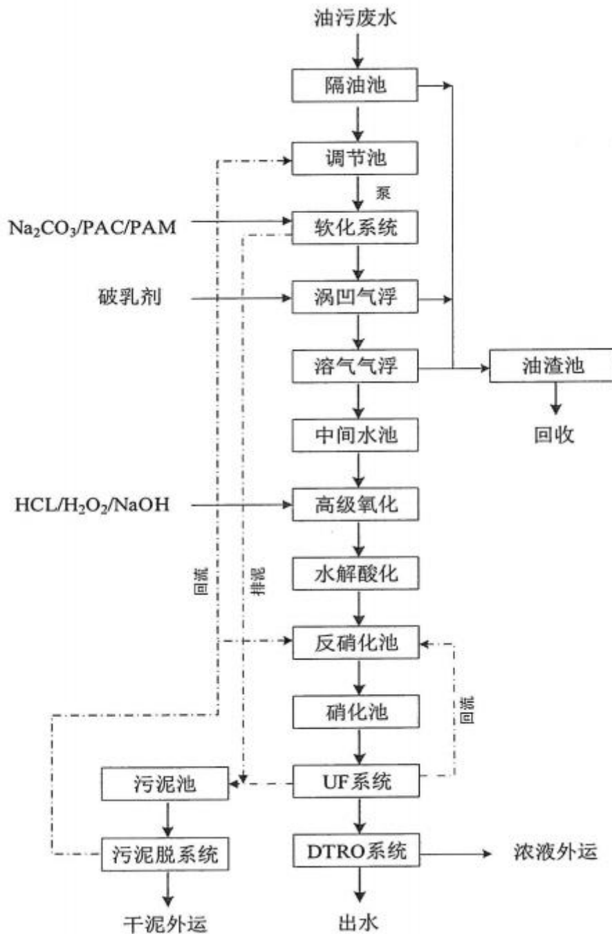
图 6.3-1 废水处理工艺流程图
