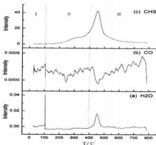
图 3.4-5 油泥在氮气下 CH 4 /CO/H 2 O 温度变化图
