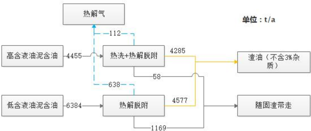
图 3.9-2 本项目油平衡图
