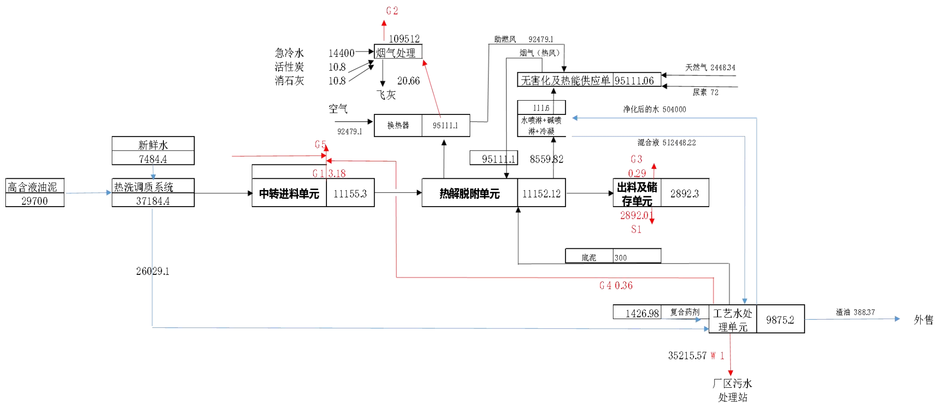
图 3.9-1 本项目全厂物料平衡图
