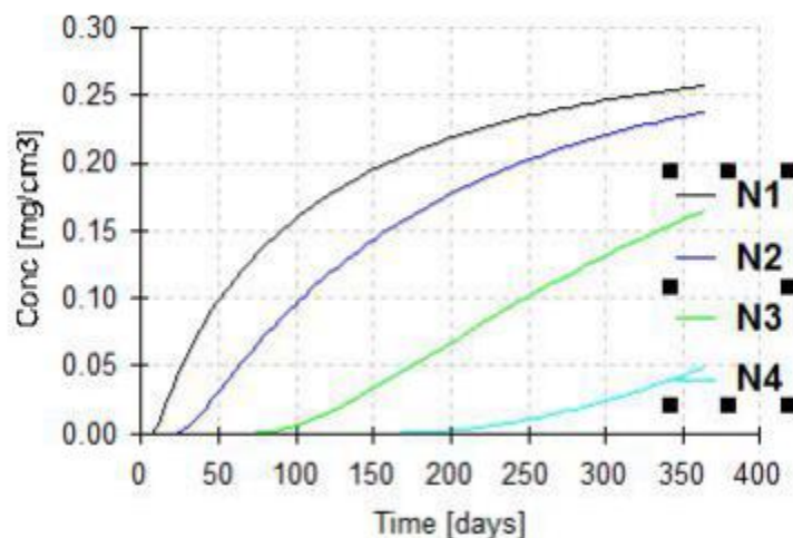
图 5.6-1 时间与浓度图
