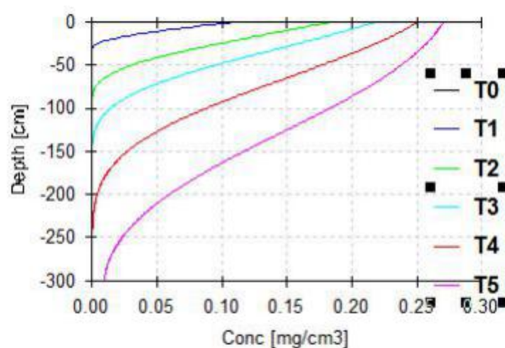
图 5.6-2 浓度与深度图
