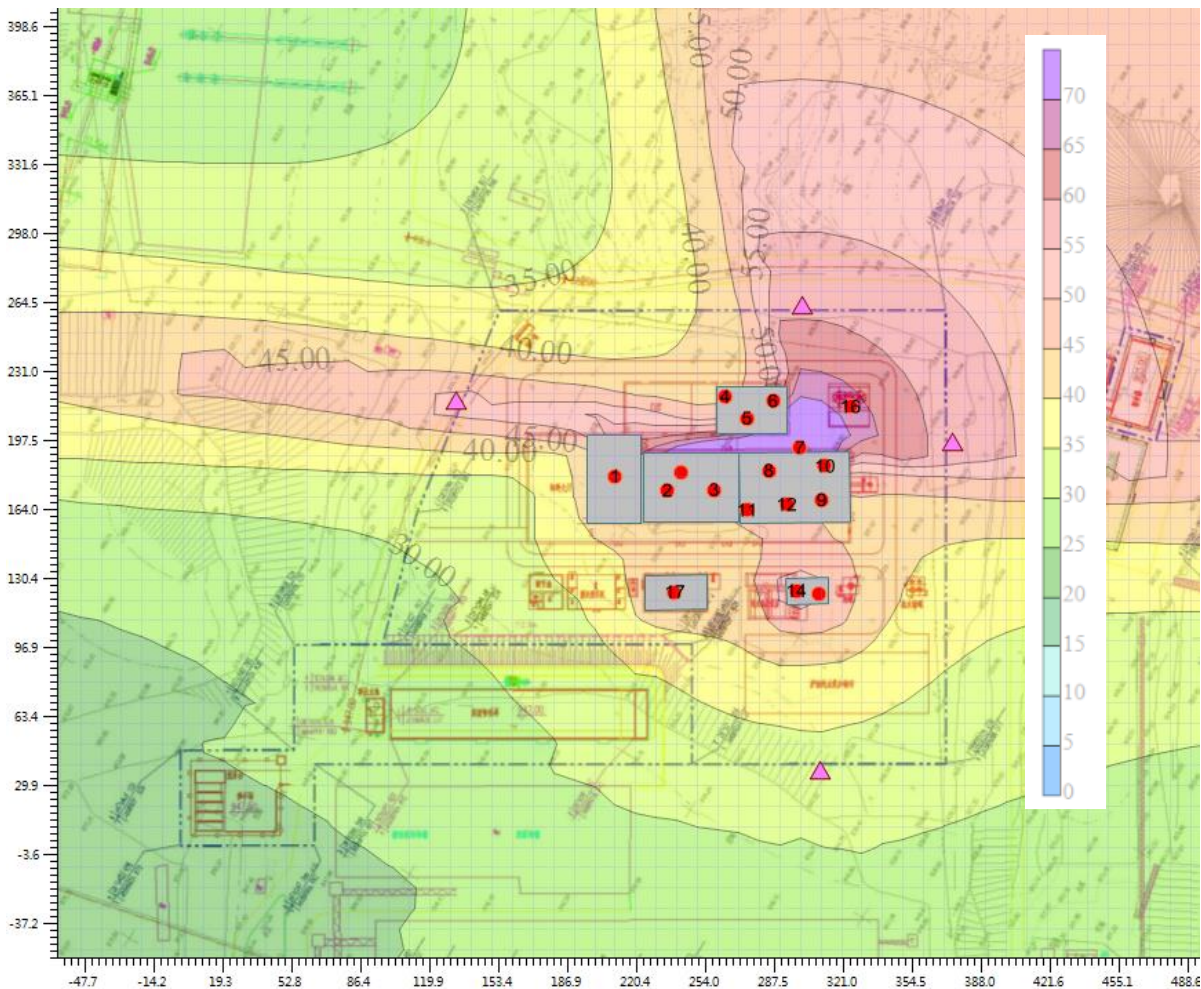
图 7.5-3 非正常工况时噪声预测等值线图
