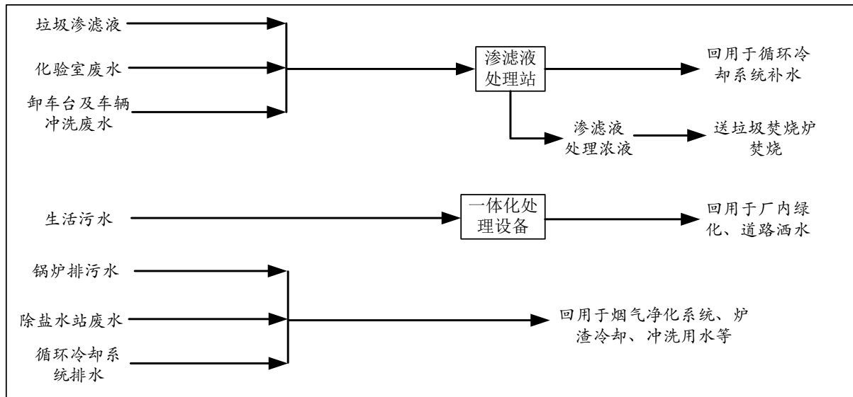
图 9.2-1 拟建项目废水污染防治措施示意图
