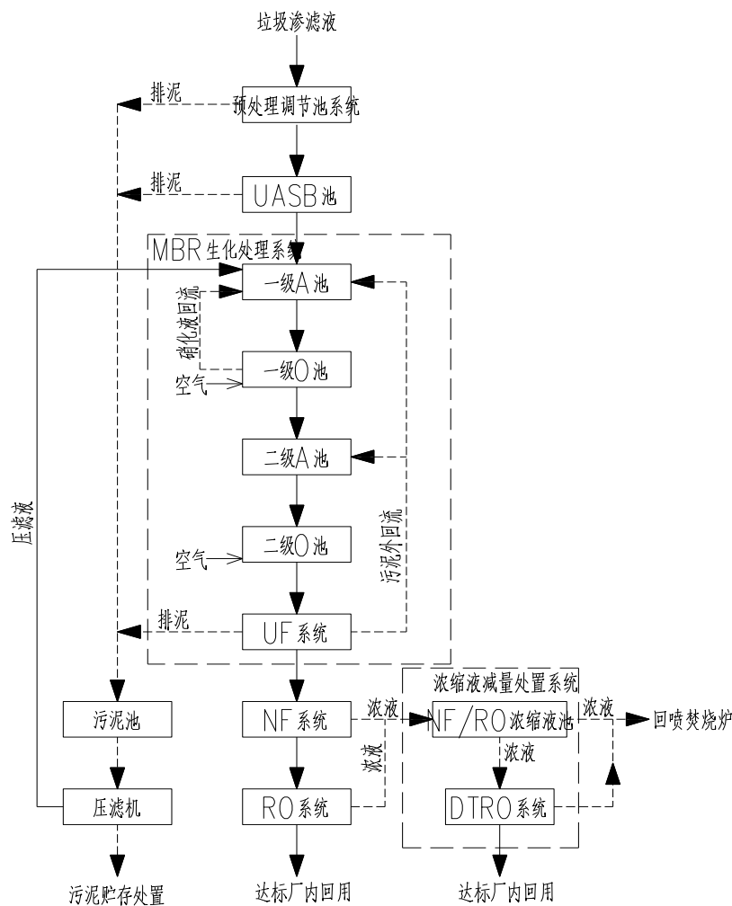
图 3.8-5 渗滤液处理系统的工艺流程图
