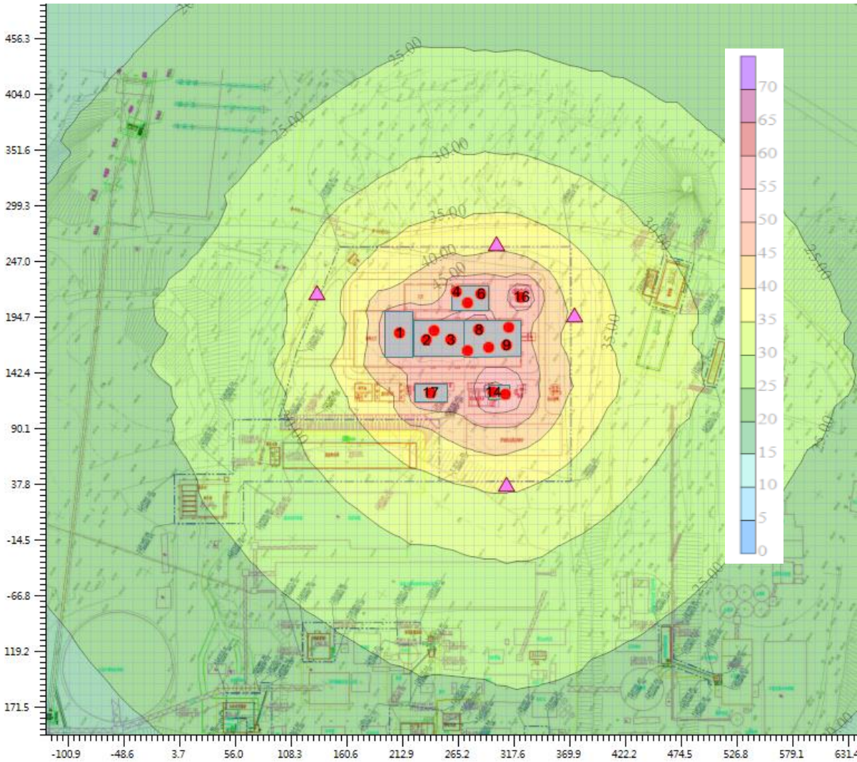
图 7.5-2 正常工况时噪声预测等值线图
