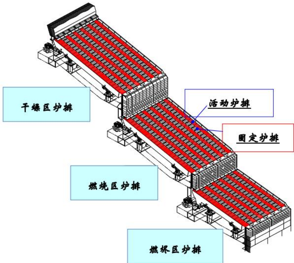
图 3.8-4 焚烧炉炉排结构示意图
